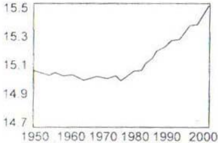
სურ. 2. საშუალო ტემპერატურის ცვლილების გლობალური ტენდენცია XX საუკუნის II ნახევარში, აკიმოვის და სხვ. (2001) მიხედვით
