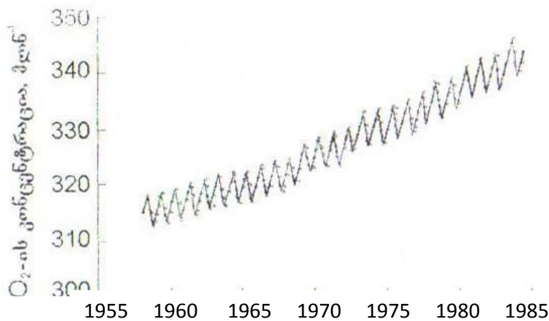
სურ. 1. \text{CO}_2 -ის კონცენტრაციის ცვლილება ატმოსფეროში (ჰავაის კუნძულების ერთ-ერთი ობსერვატორიის მონაცემები, გ. ქაჯაია, 2008)
